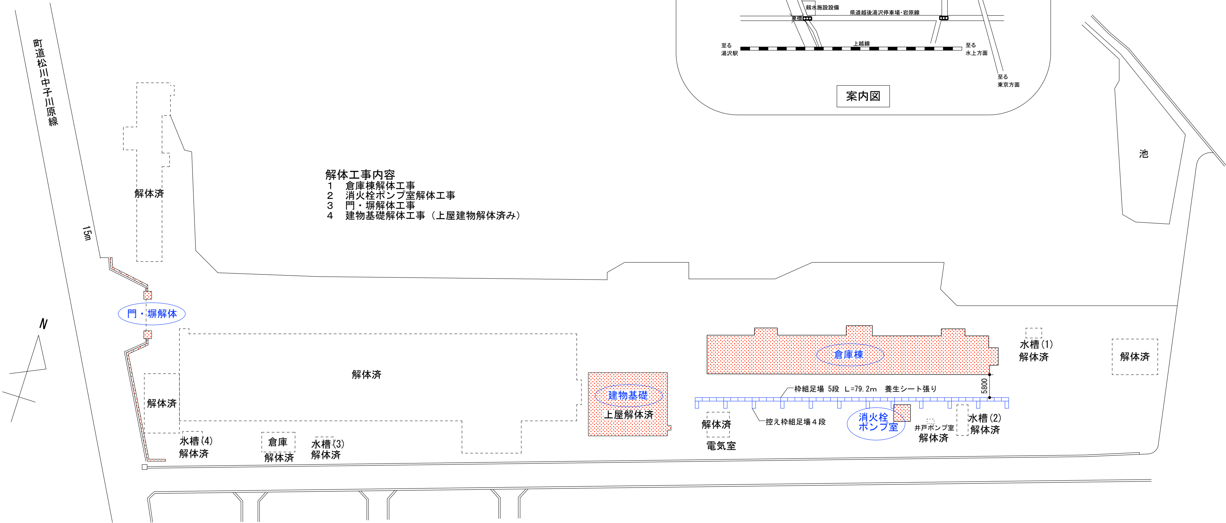
配置図 S=1 : 600
