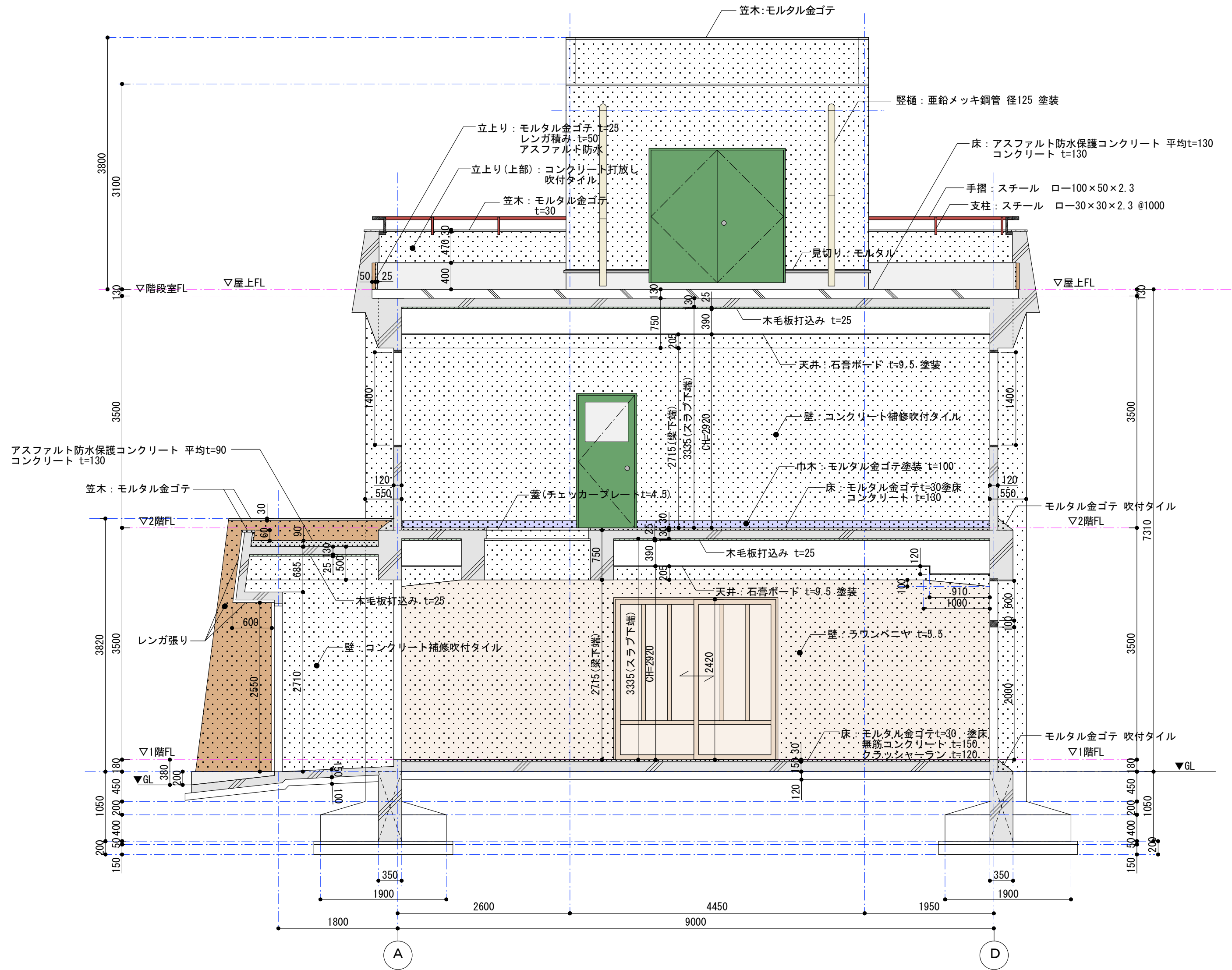
断面詳細図 S=1 : 50
