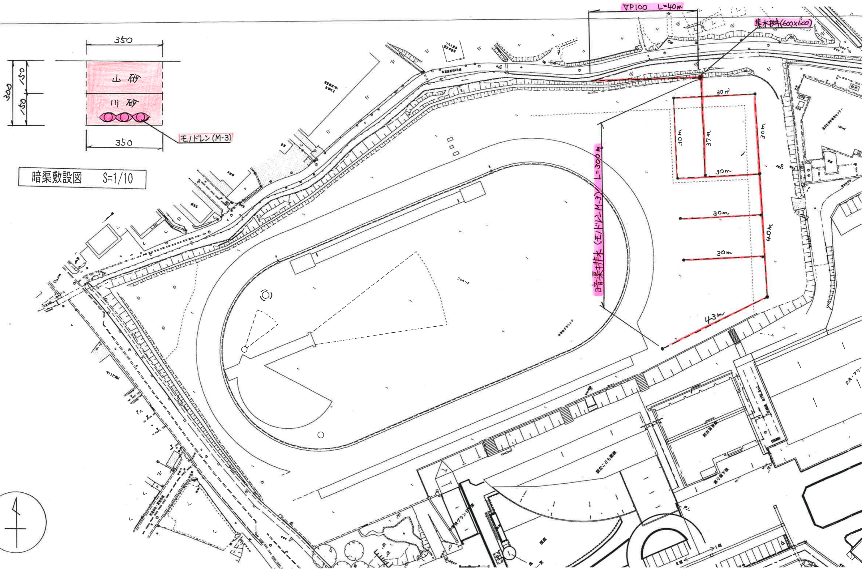
学工第1号 湯沢学園野球場排水施設工事 S=1:800
