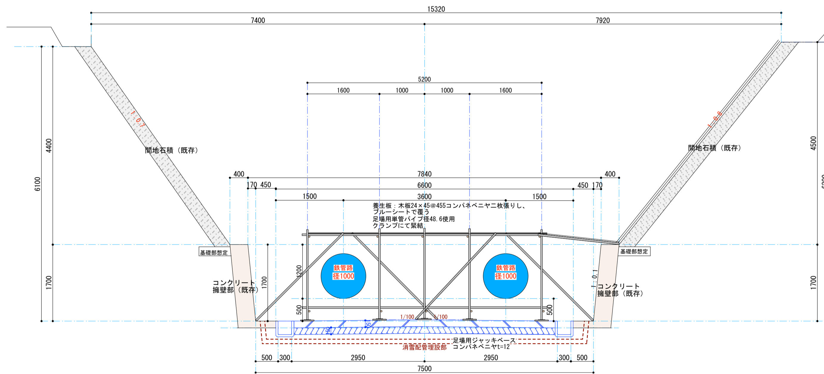
A-A断面
