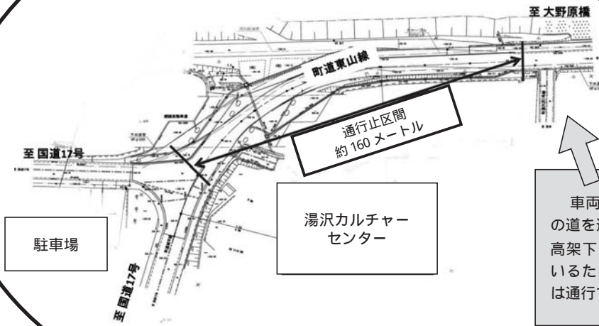
工事場所位置図
