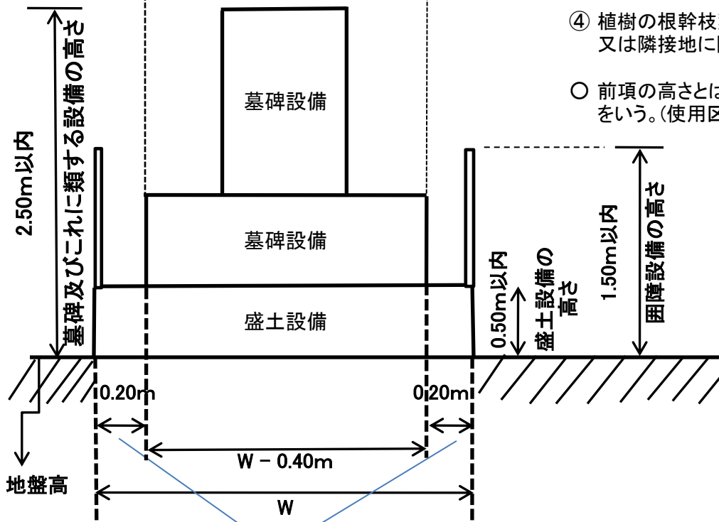
断面図
